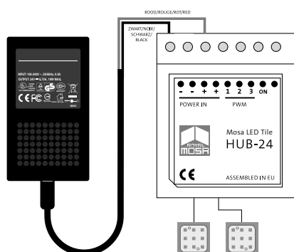
EV10WHB000005 elektronische voeding 100/240V AC 24V/10W plus connectionbox voor maximaal 5 aansluitingen / alimentation électronique 100 / 240V AC 24V / 10W et boîte de connexion pour maximum 5 raccordements / Trafo 100/240V AC 24V/10W plus Anschlusskasten für bis zu 5 Anschlüsse / electronic 100/240V AC power supply 24V/10W plus connectionbox for a maximum of 5 connections
