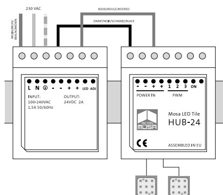
EV45WHB000024 elektronische voeding 100/240V AC 24V/45W plus connectionbox voor maximaal 24 aansluitingen / alimentation électronique 100 / 240V AC 24V / 45W et boîte de connexion pour maximum 24 raccordements / Trafo 100/240V AC 24V/45W plus Anschlusskasten für bis zu 24 Anschlüsse / electronic 100/240V AC power supply 24V/45W plus connectionbox for a maximum of 24 connections
